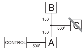
Diagrama 2-2: Cableado Corbus
