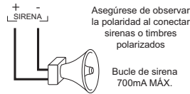
Diagrama 2-12: Cableado de terminales Timbre
