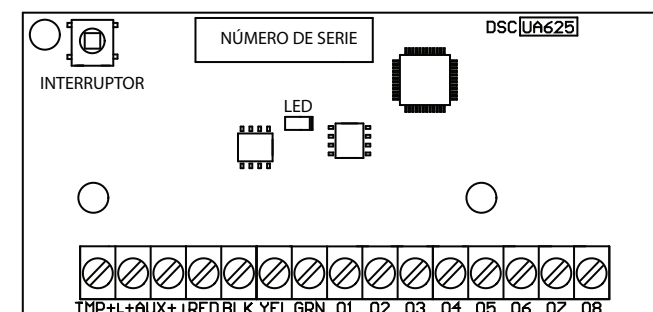
Diagrama 2-4: HSM2208 Expansor de salida
