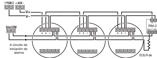
Diagrama 2-14: Cableado del detector de humo
