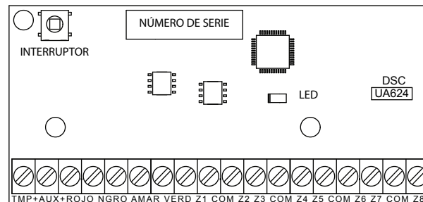
Diagrama 2-3: HSM2108 Expansor de zona
