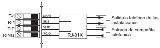
Diagrama 2-13: Cableado de línea telefónica
