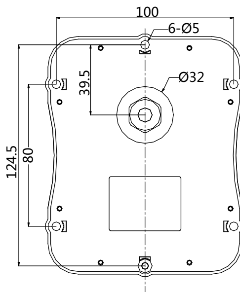
Vista trasera
