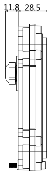
Vista lateral
