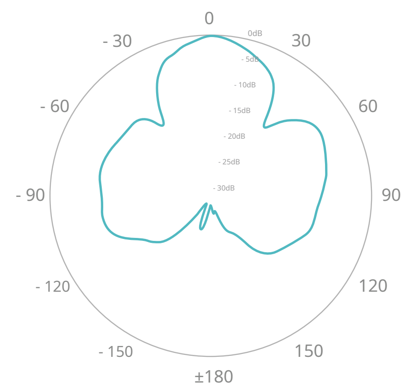
Elevación horizontal
