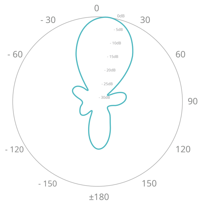
Elevación horizontal
