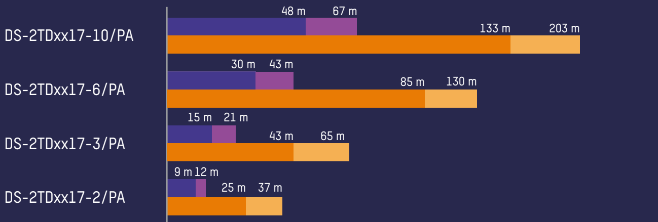
Distancia para la detección VCA de personas o vehículos
